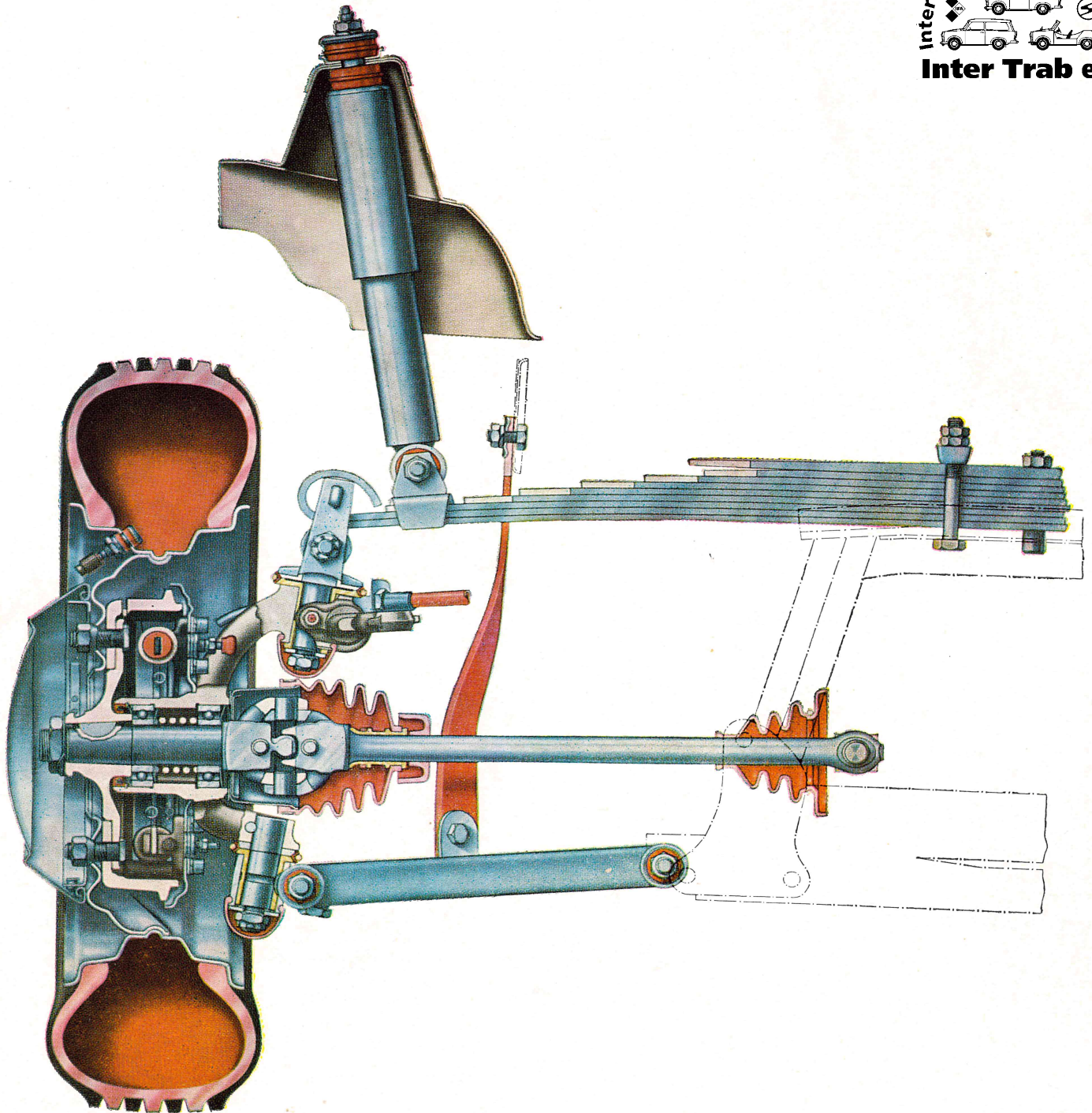
Bild F 10. Radantrieb – Schnitt
